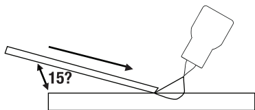
Add Tig filler wire
